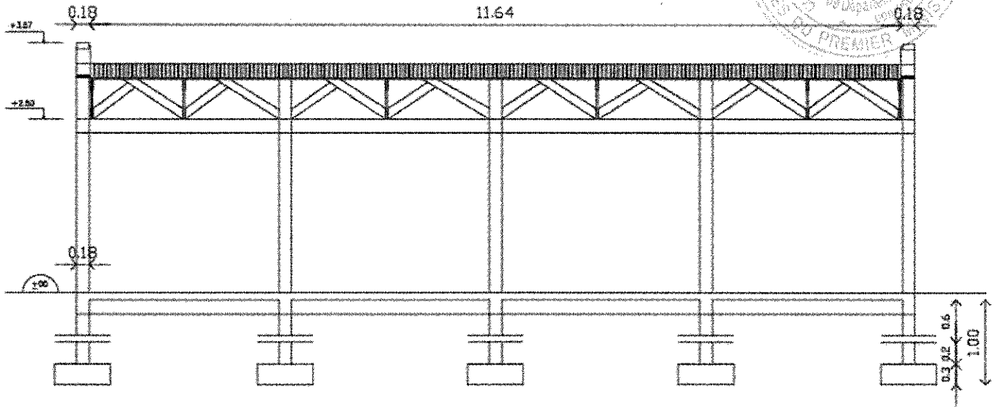
COUPE B-B
